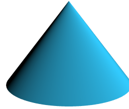
Cone
